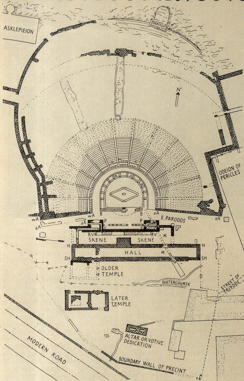
Σχεδιάγραμμα του θεάτρου που έντοπίζει τίς διαδοχικές φάσεις των ύπολειμμάτων.
